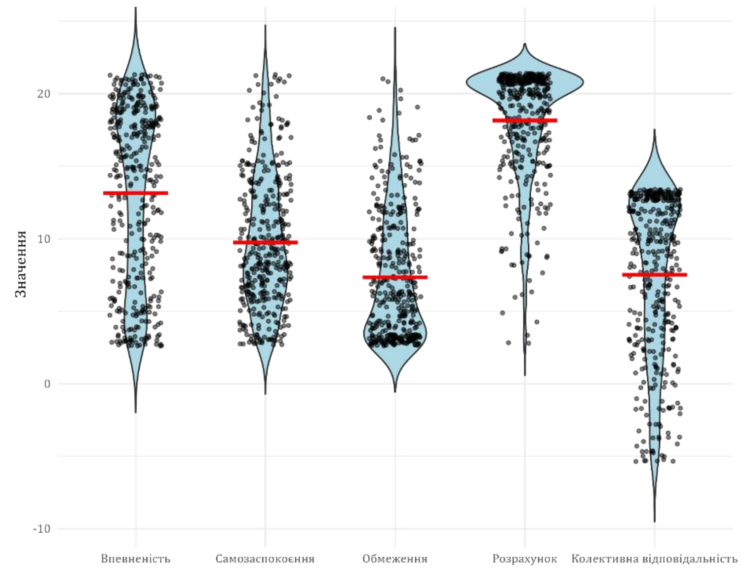
Рис. 1. Розподіл отриманих значень за кожною субшкалою «5С Психологічні передумови вакцинації» із позначенням середнього значення
