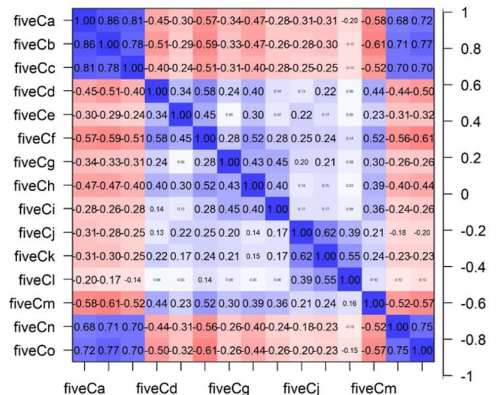
Рис. 5. Факторна структура «Шкали хемофобії» (двофакторне рішення)
