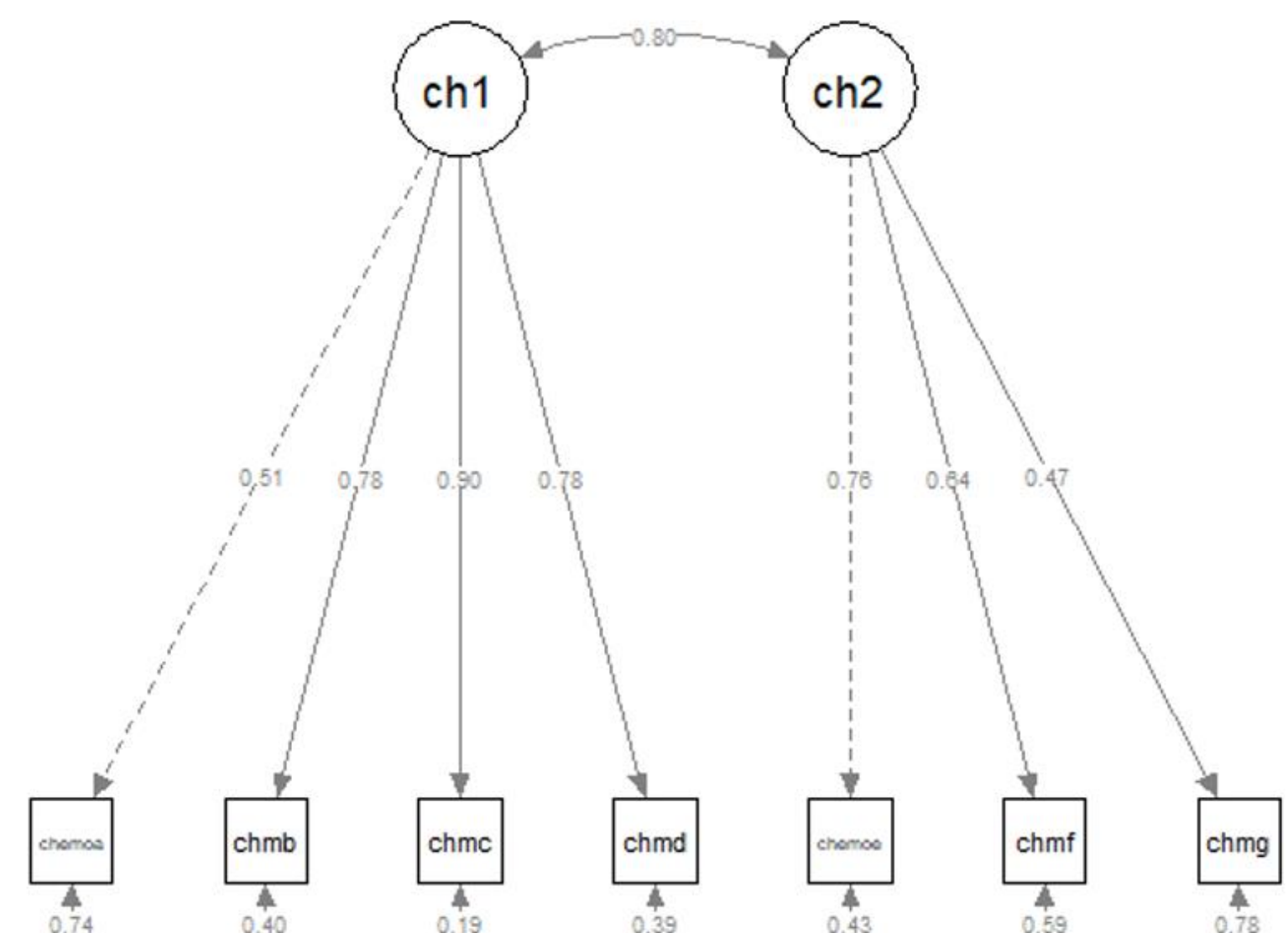
Рис. 5. Факторна структура «Шкали хемофобії» (двофакторне рішення)
