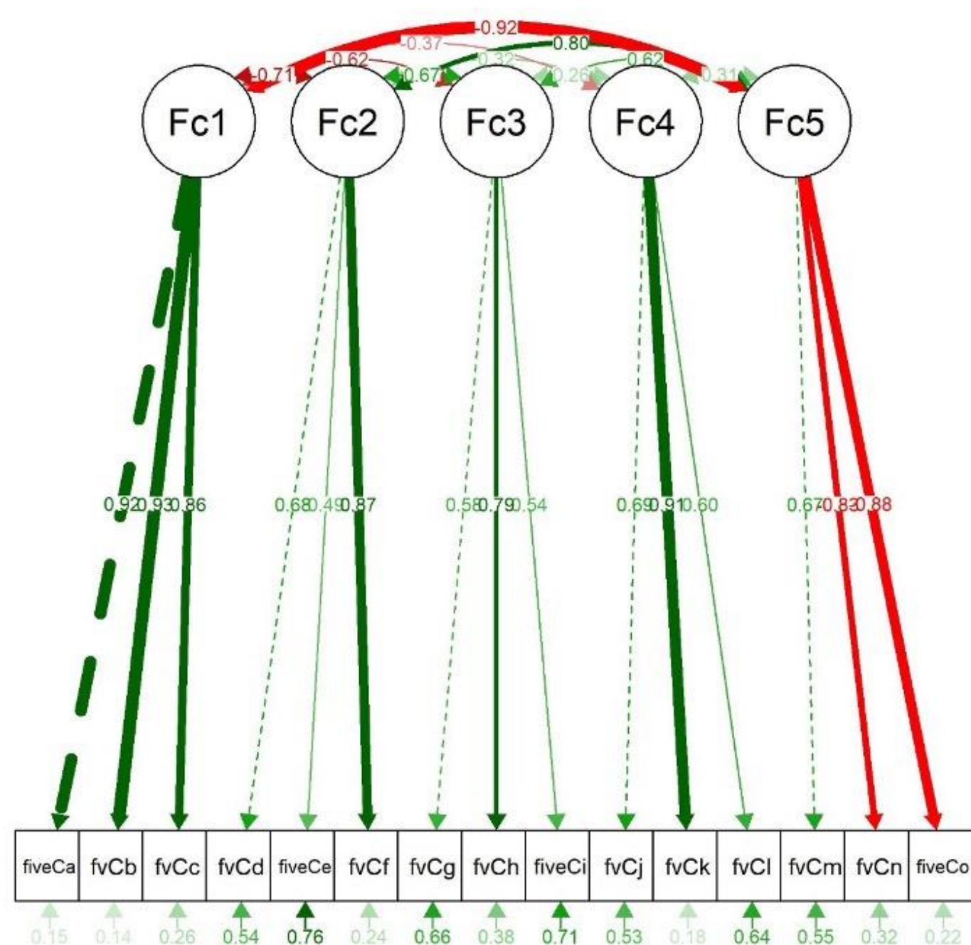
Рис. 4. Факторна структура «Багатовимірної шкали локусу контролю здоров'я»
