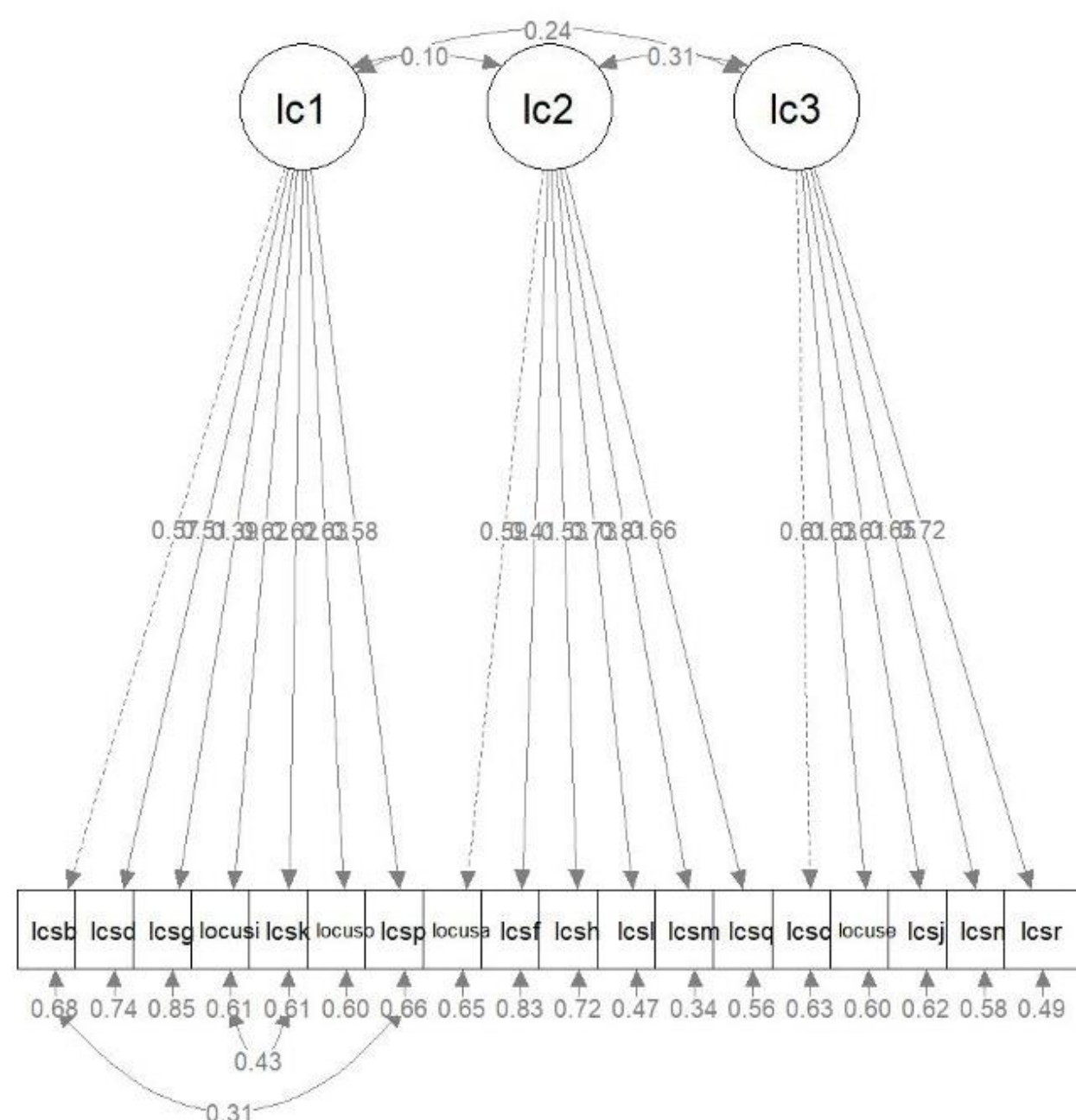
Рис. 4. Факторна структура «Багатовимірної шкали локусу контролю здоров'я»
